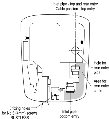
Fig. 6 Template schematic
