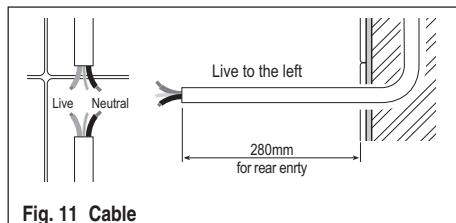
Fig. 11 Cable
