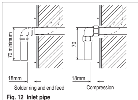
Fig. 12 Inlet pipe
